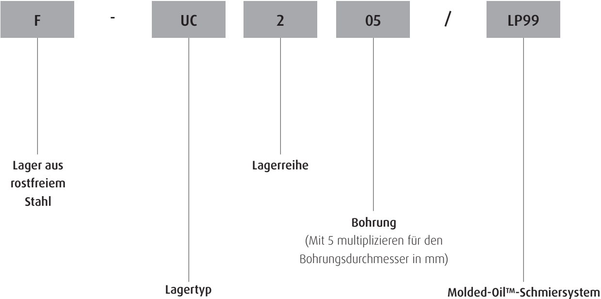
Molded-Oil™-Lagereinsatz Bezeichnungssystem
