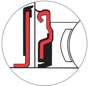
Einlippendichtung + Schleuderscheibe
