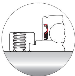
Exzenterring
