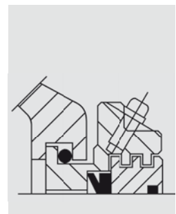
TACK-Dichtungen
