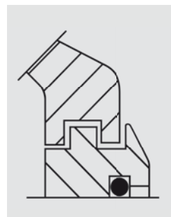
TS-U-Dichtungen
