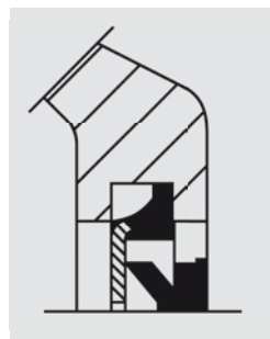
V-Dichtungen
