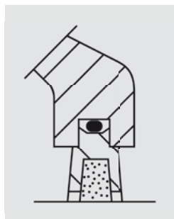
C-Dichtungen
