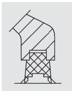
G-Dichtungen
